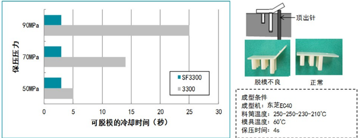
图2-1 SF3300与3300的脱模性比较
