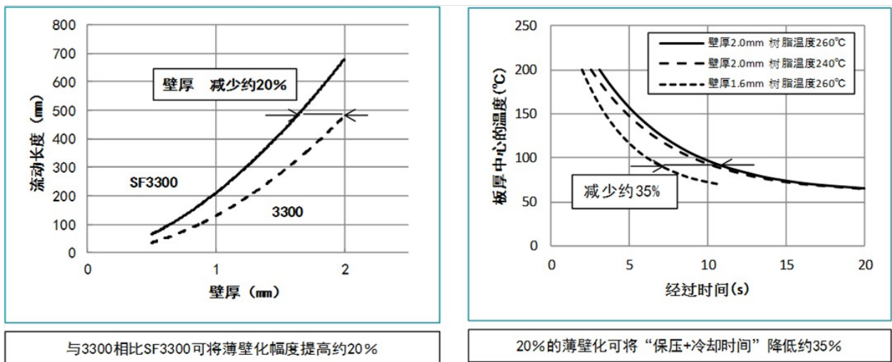
图2-2 高流动性与薄壁化
